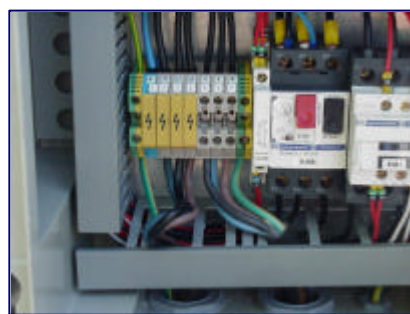
Branchement électrique sur bornier
